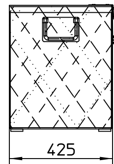
Ansicht links Maßstab 1:15
