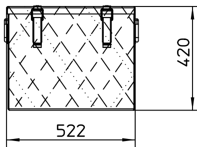
AllgSicht Maßstab 1:15
