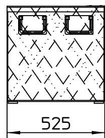
Ansicht links
